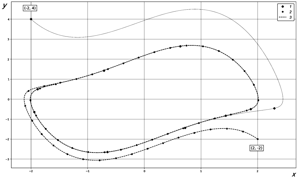
Рис. 1. Тренировочные данные, сгенерированные при (x_0, y_0) = (-2, 4) (1), тестовые данные, сгенерированные при (x_0, y_0) = (2, -2) (2), и спрогнозированные на тестовых значения с помощью построенной модели динамической полиномиальной регрессии (3)
